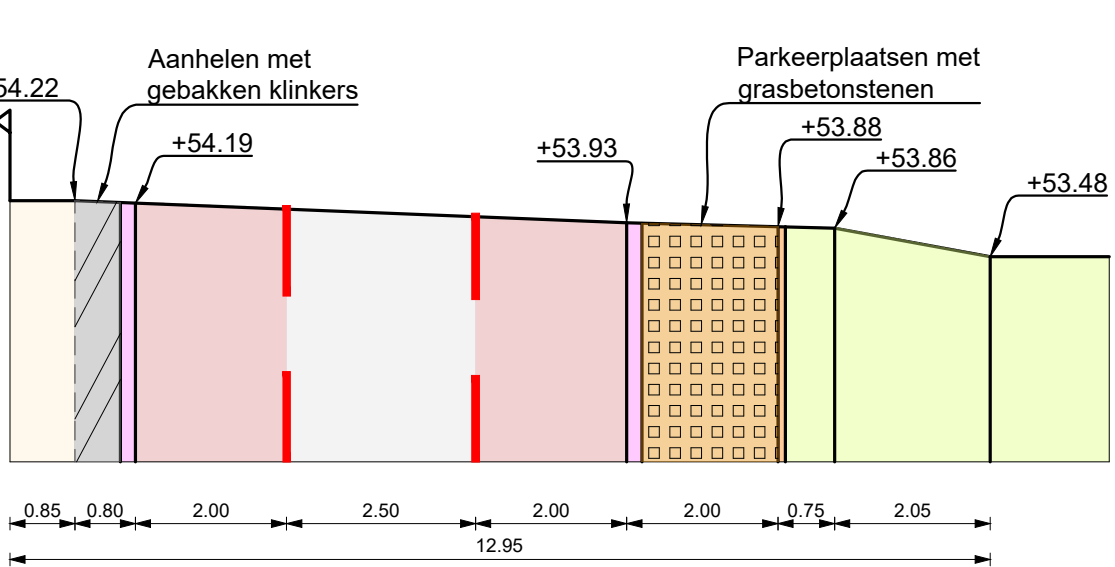
Dwarsprofiel C - C nieuwe situatie
