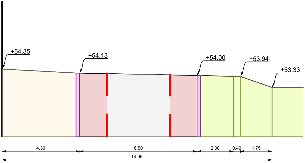
Dwarsprofiel B - B bestaande situatie
