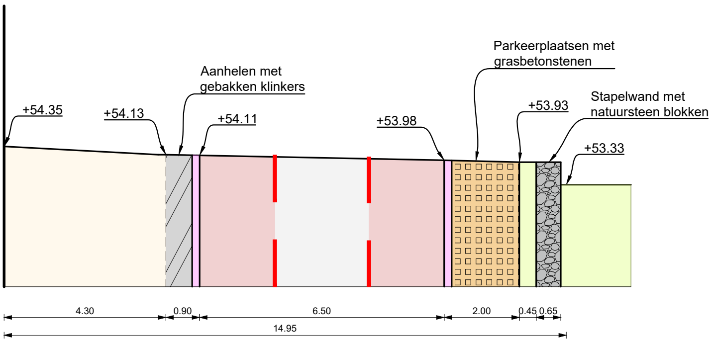
Dwarsprofiel B - B nieuwe situatie
