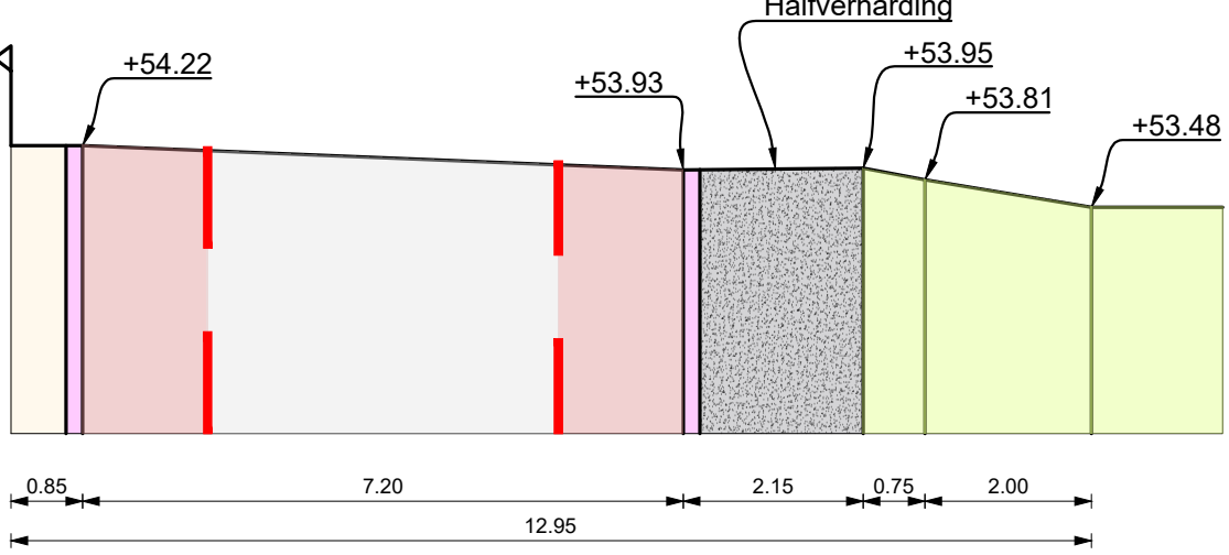
Dwarsprofiel C - C bestaande situatie
